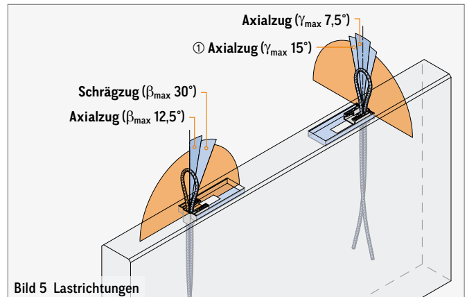
Bild 5 Lastrichtungen
