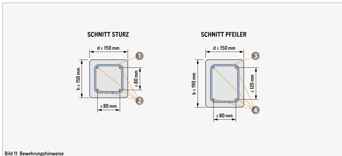
Bild 11 Bewehrungshinweise
