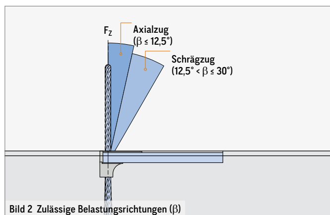
Bild 2 Zulässige Belastungsrichtungen ( \beta )
