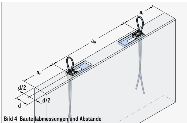
Bild 4 Bauteilabmessungen und Abstände
